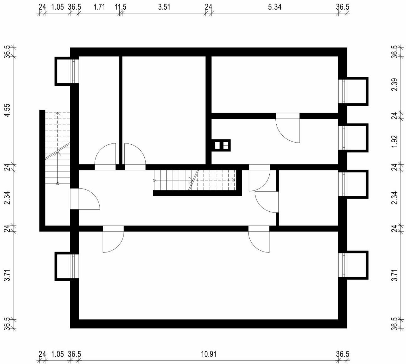
Kellergeschoss
