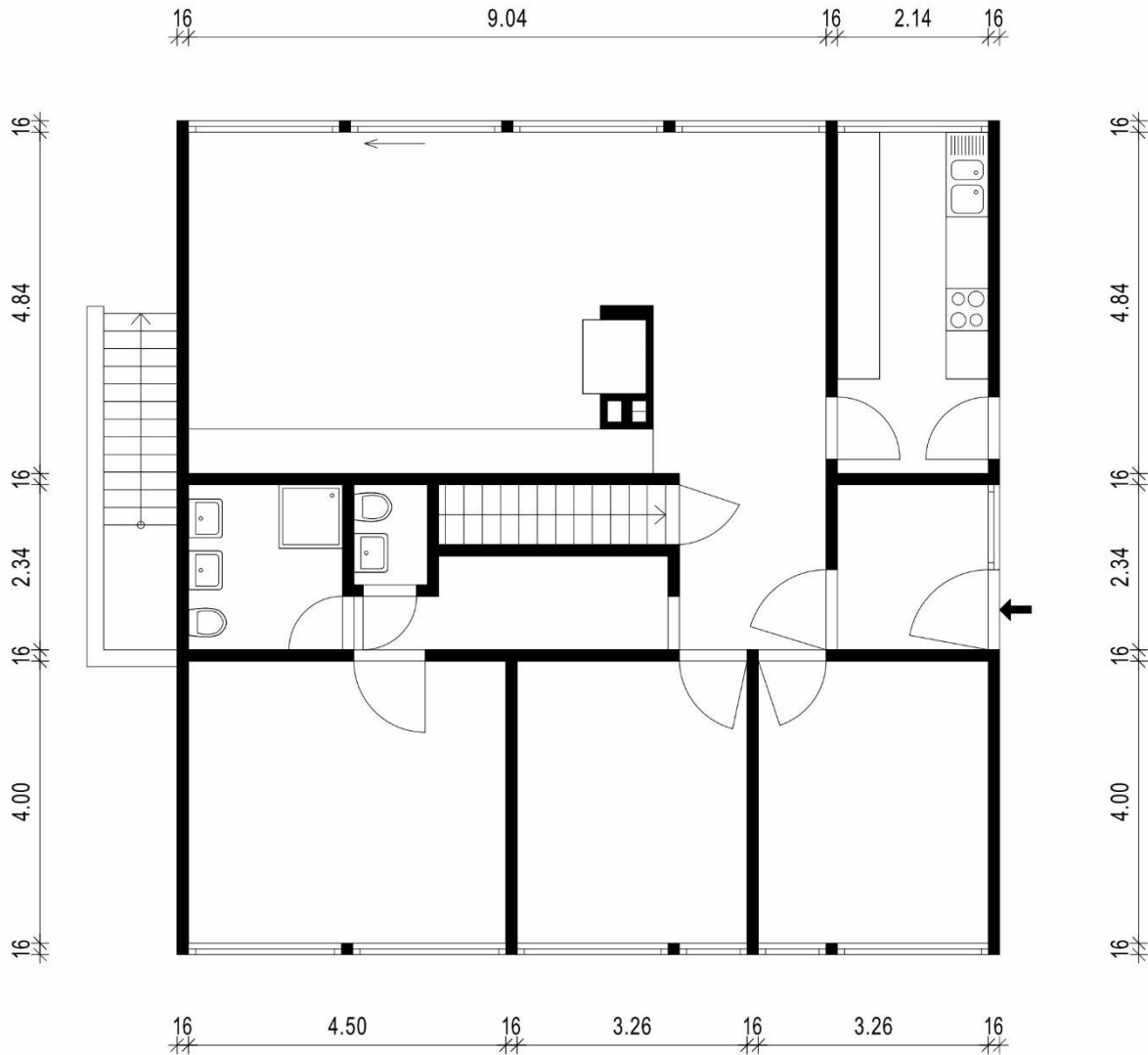
Erdgeschoss
